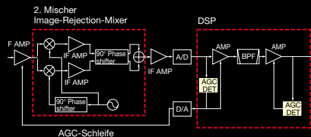
DIGI-SEL-Einheit
