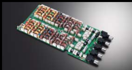
Bandpassfilter-Einheit
